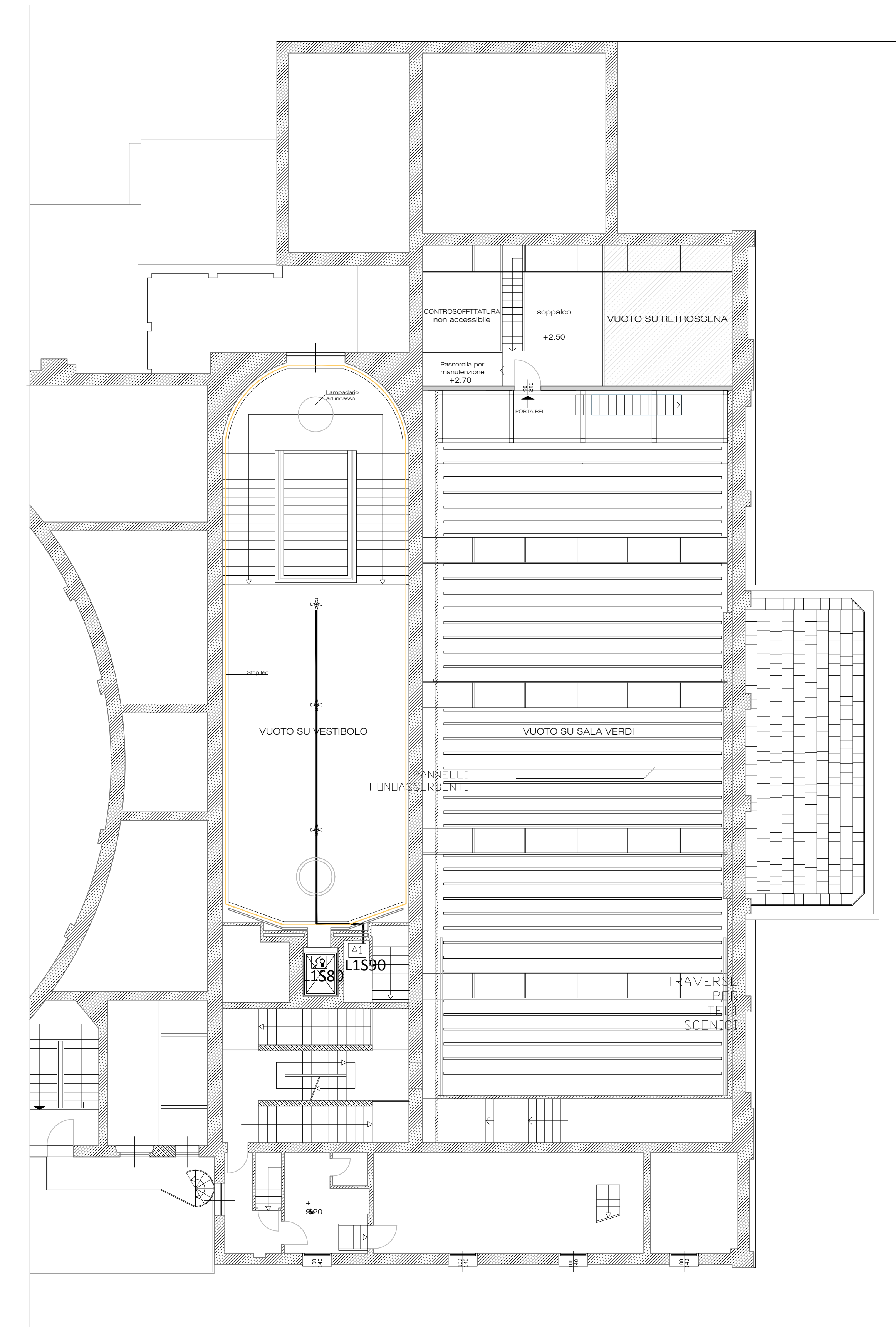
PIANTA SALA VERDI - QUOTA +9.20
