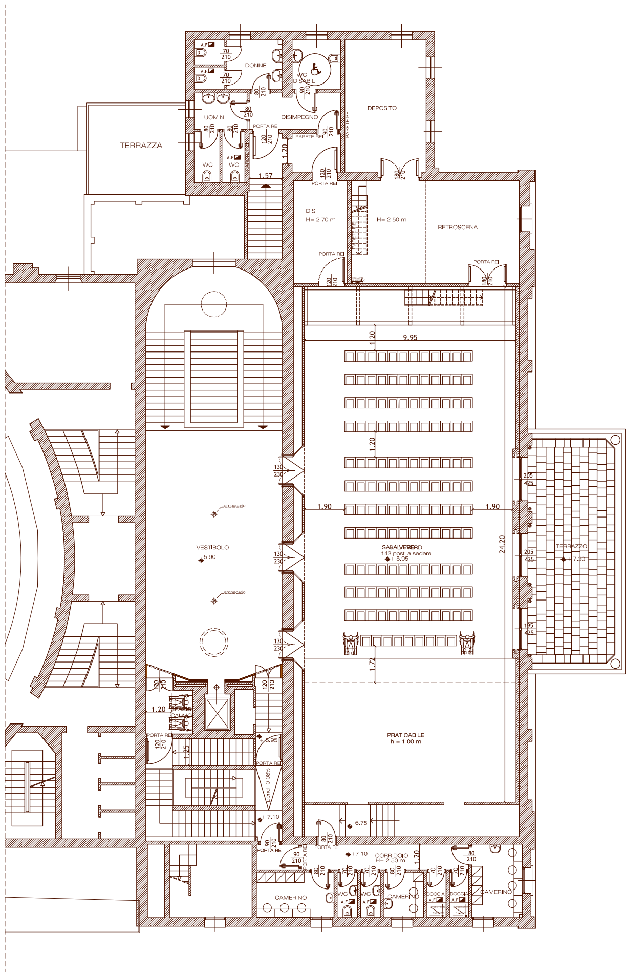
PIANTA PIANO PRIMO soluzione palcoscenico
