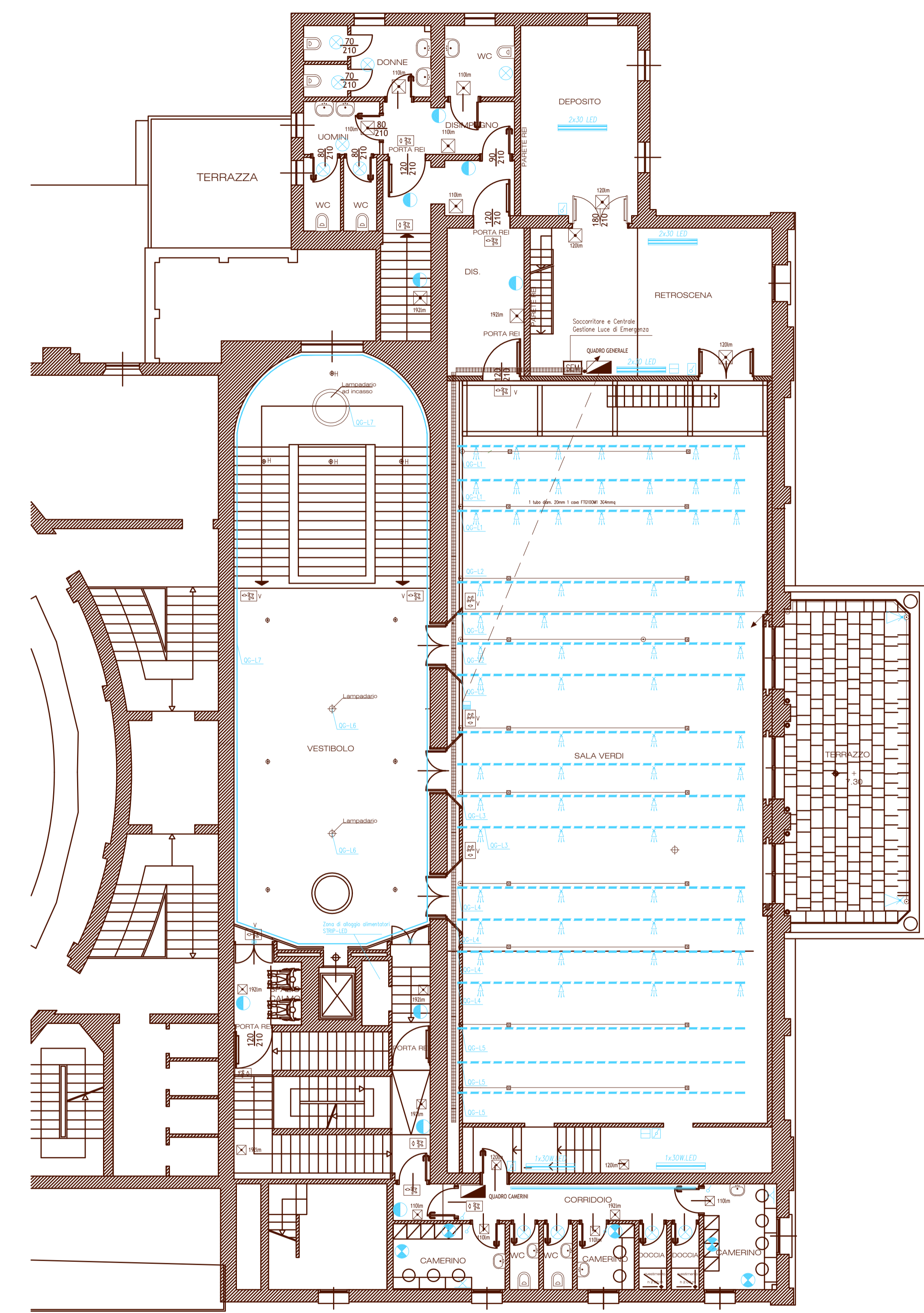
PIANTA PIANO PRIMO LUCE SCALA 1:100
