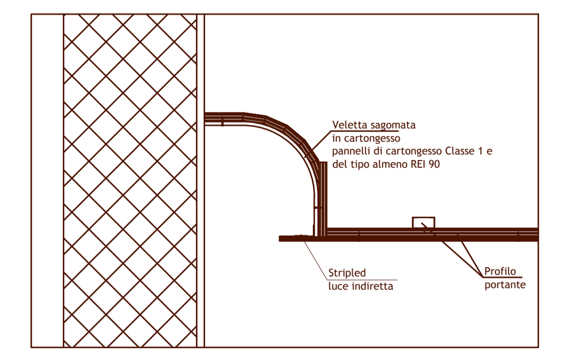
PARTICOLARE CONTROSOFFITTO IN CARTONGESSO CON LUCE PERIMETRALE (FUORI SCALA)
